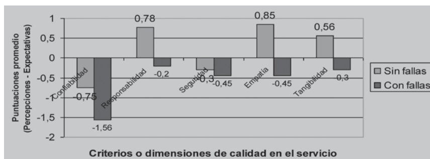
Gráfico 3 >>> Puntuación de Servqual por dimensiones y por grupos de clientes que percibieron y no percibieron fallas en el servicio.
