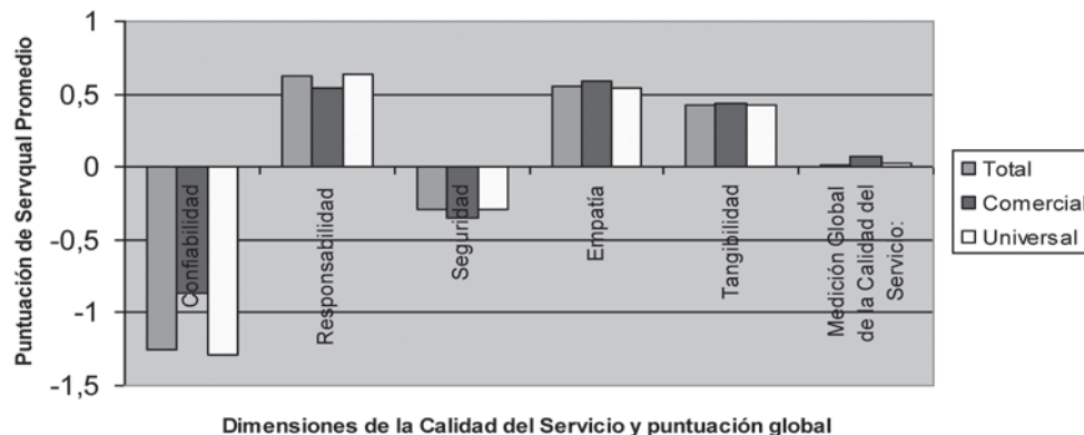
Gráfico 2 >>> Puntuaciones Global de Servqual, por criterio de calidad en el servicio y por tipo de banca.
