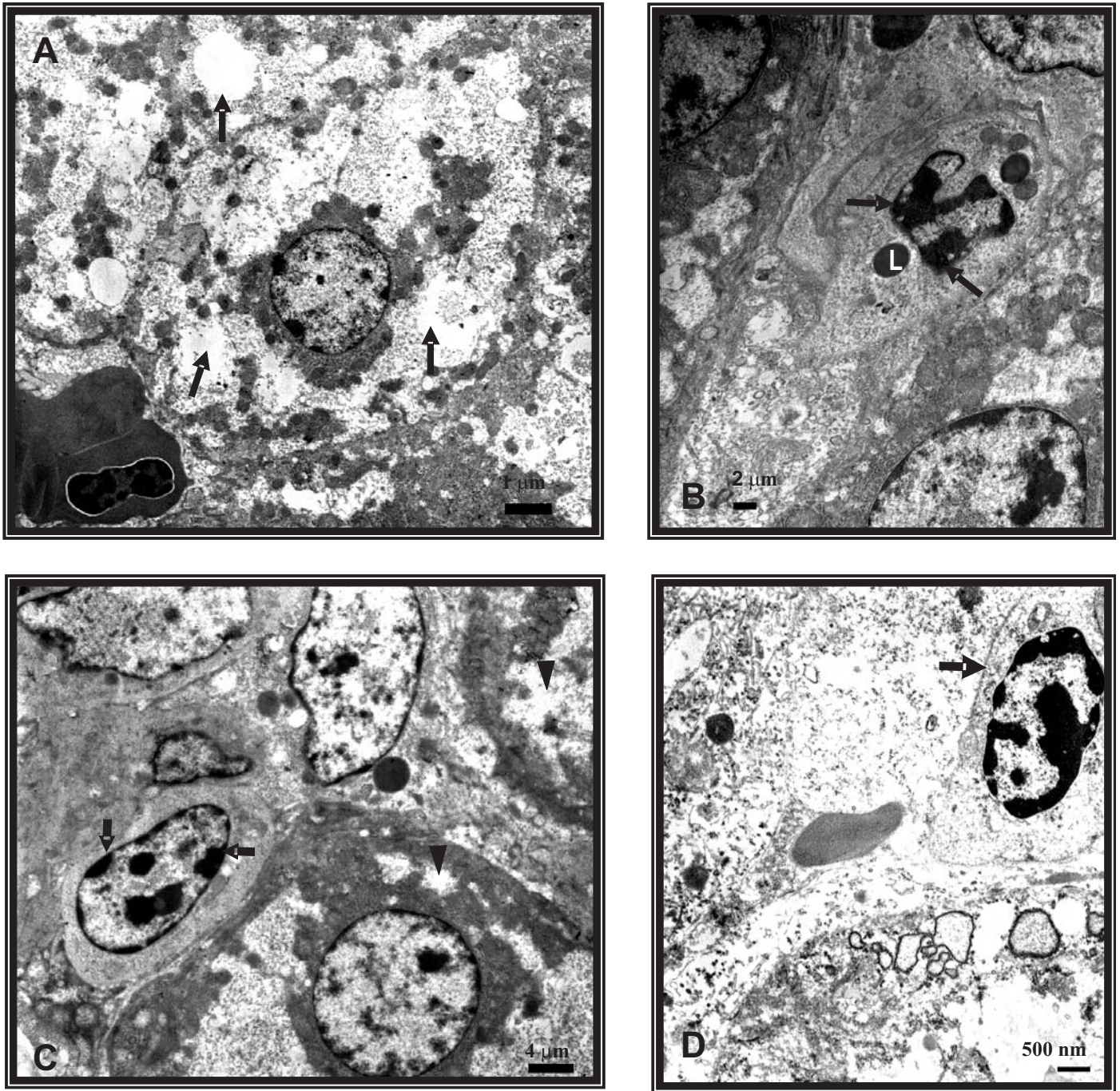
FIGURA 3. A) DIETA CON Sc + AFB 1 (T 4 ). ZONA DE LISIS INTRACITOPLASMÁTICA (↑) EN UN HEPATOCITO. 10.000X. B) DIETA CON AFB 1 (T 2 ). CÉLULA CON CONDENSACIÓN DE LA CROMATINA NUCLEAR (↑), DONDE SE OBSERVA DOS VACUOLAS DE LÍPIDO (L). 8.000X. C) DIETA CON Se + AFB 1 (T 6 ). PANORÁMICA MOSTRANDO SINUSOIDE HEPÁTICO CON POSIBLES CÉLULAS SANGUÍNEAS MONONUCLEARES, CON CONDENSACIÓN NUCLEAR (↑) SUGERENTES APOPTOSIS Y ZONAS DE LISIS CITOPASMÁTICAS (▲) 5.000X. D) DIETA CON Sc + Se + AFB 1 (T 8 ). PANORÁMICA MOSTRANDO CÉLULAS EN LISIS Y CÉLULA APOPTÓTICA (↑) 10.000X. / A) FED WITH Sc + AFB 1 (T 4 ). OBSERVE INTRACYTOPLASMIC LYSIS ZONES (↑) IN A HEPATOCYTE LINING A HEPATIC SYNUSOID WHERE AN ERYTHROCYTE IS SEEN (e). 10.000X. B) RATION CONTAINING AFB 1 (T 2 ). CELLS WITH NUCLEAR CHROMATIN CONDENSATION (↑), WHERE TWO LIPID VACUOLES ARE OBSERVED (L). 8.000X. C) FED WITH Se + AFB 1 (T 6 ). LOW ZOOMED SHOT SHOWING A HEPATIC SYNUSOID WITH POSSIBLE MONONUCLEAR BLOOD CELLS, WITH NUCLEAR CONDENSATION (↑) SUGGESTING APOPTOSIS AND CYTOPLASMIC LYSIS (▲) 5.000X. D) FED WITH Sc + Se + AFB 1 (T 8 ). LOW ZOOMED SHOT SHOWING LYSED CELLS AND APOPTOTIC CELL (↑) 10.000X. (AFB 1 = Aflatoxina B 1 ; Sc= cultivo de S. cerevisiae ; Se= Selenio).
