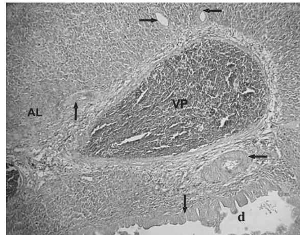
FIGURA 2. ESPACIOS PORTALES ENGROSADOS CON PROLIFERACIÓN DE CONDUCTOS BILIARES (↑), DILATACIÓN (d), CONGESTIÓN DE VENA PORTA (VP) Y AGREGADOS LINFÓCIDOS (AL). HEMATOXILINA-EOSINA 170X./ NOTE THICKENING OF PORTAL SPACES WITH BILE DUCTULE PROLIFERATION (↑), AND DILATATION (d), CONGESTION OF THE PORTAL VEIN (VP), AGGREGATES OF LYMPHOCYTES (AL). HAEMATOXYLIN-EOSIN 170X.
