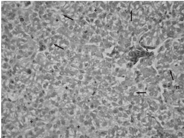
FIGURA 1. LESIÓN HEPATOTÓXICA MODERADA (LHTM). OBSÉRVESE HEPATOCITOS CON VACUOLAS LIPÍDICAS Y/O HÍDRICAS (↑), NÚCLEOS CONSERVADOS (n), NECROSIS DE HEPATOCITOS CON AUSENCIA DE NÚCLEOS (+) Y SINUSOIDES DILATADOS POR ERITOCITOS (S). HEMATOXILINA-EOSINA 680X./ MODERATE HEPATOTOXIC LESION (LHTM). NOTE HEPATOCYTES WITH LIPID AND/OR HIDRIC VACUOLES (↑), HEPATOCYTES NORMAL NUCLEI (n), HEPATOCYTES NECROSIS WITHOUT NUCLEI (+), DILATATED SINUSOIDS BY RED BLOOD CELL (S). HAEMATOXYLIN-EOSIN 680X.
